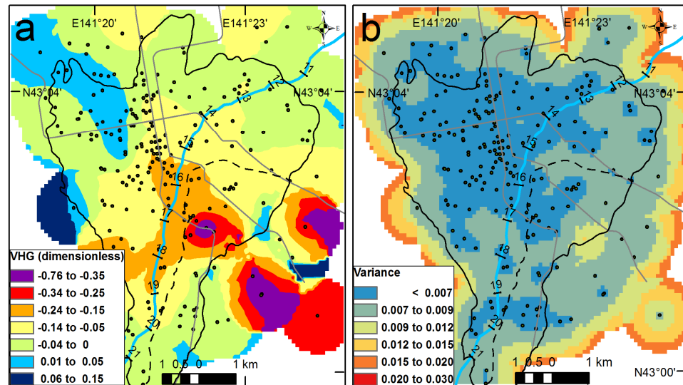
鉛直動水勾配マッピング (左: 鉛直動水勾配, 右: 推定誤差分散)
